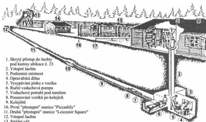
Nákres tunelu
